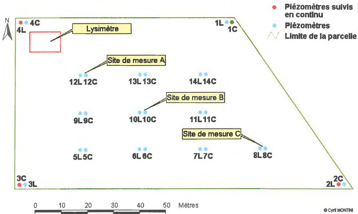
Figure 4 : Schéma de l'instrumentation du site atelier "Fontanille"
