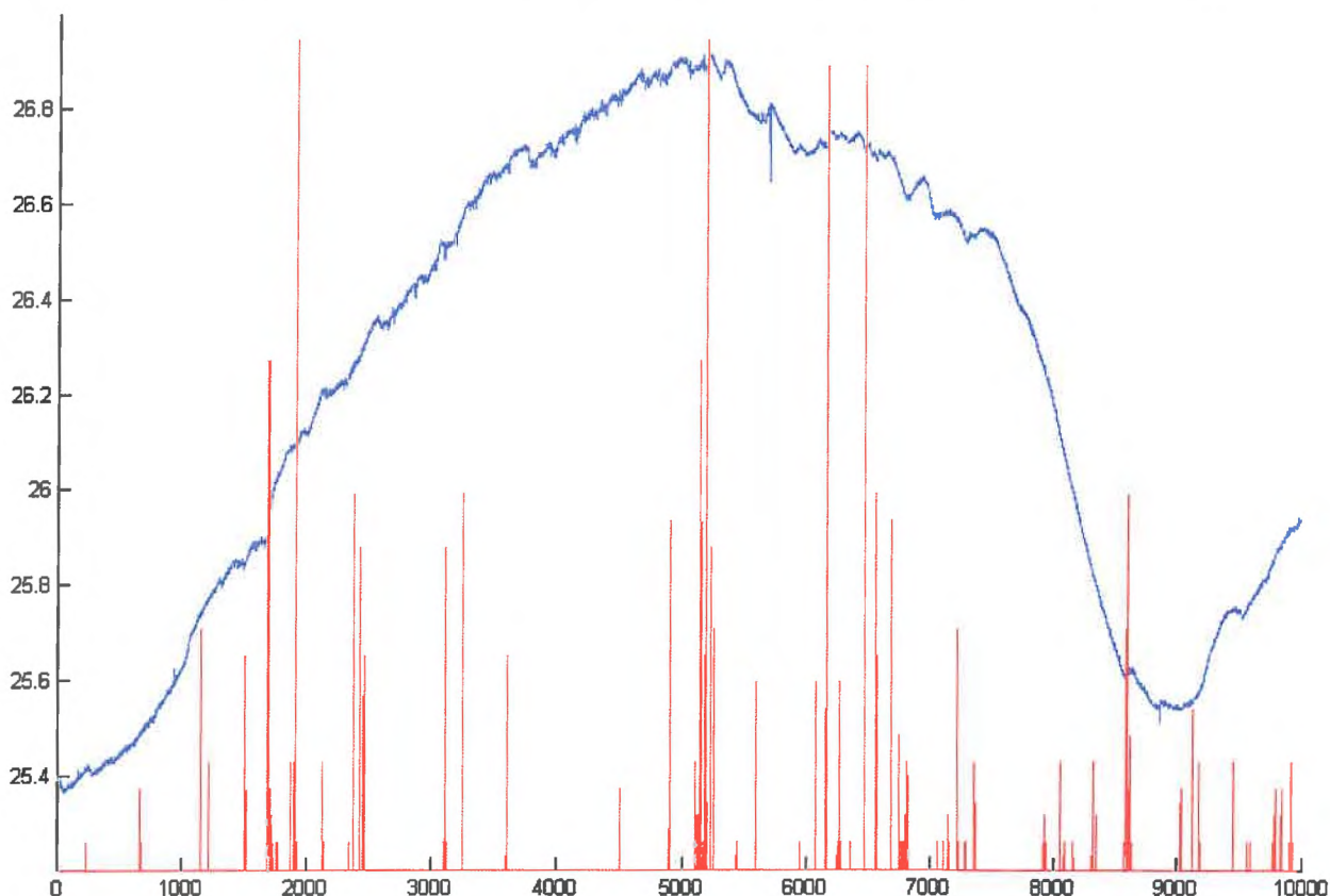
Figure 15 : Signal piézométrique brut avec la chronique de pluie
