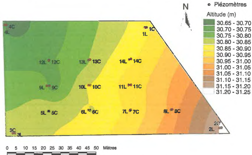
Figure 3 : Modèle Numérique de Terrain (MNT) du site atelier "Fontanille"
