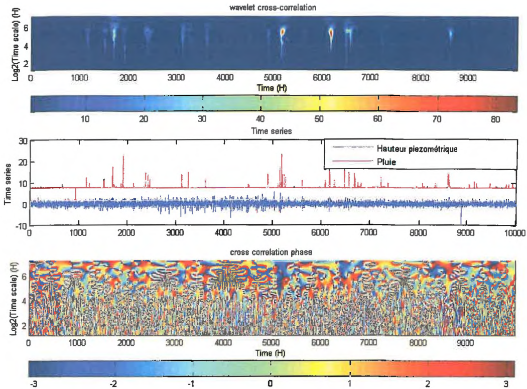
Figure 19 : Corrélation croisée entre le signal des fluctuations et le signal de pluie
