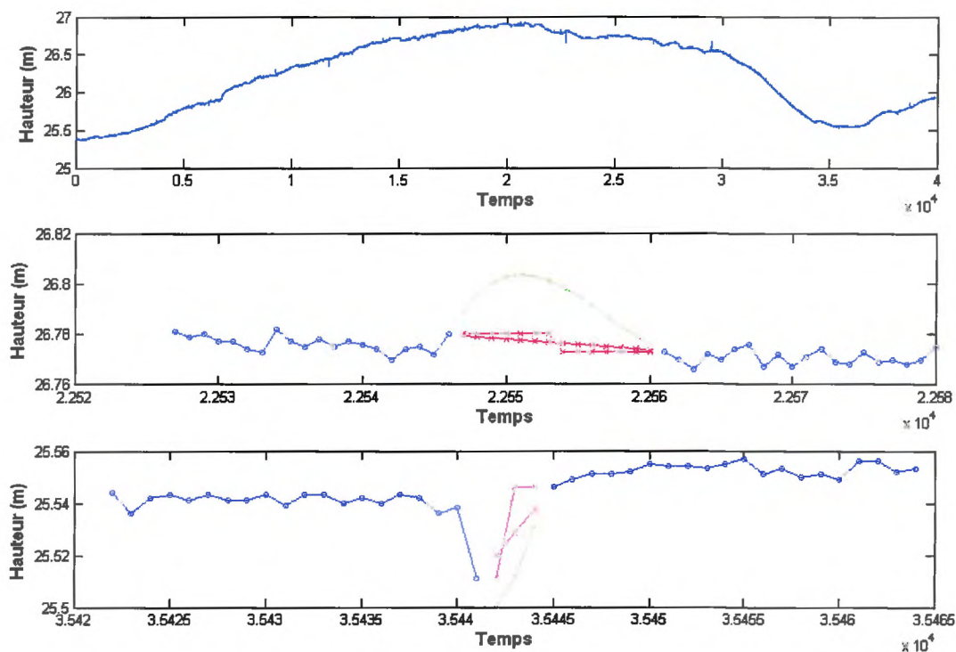
Figure 14 : Interpolation du signal piézométrique
