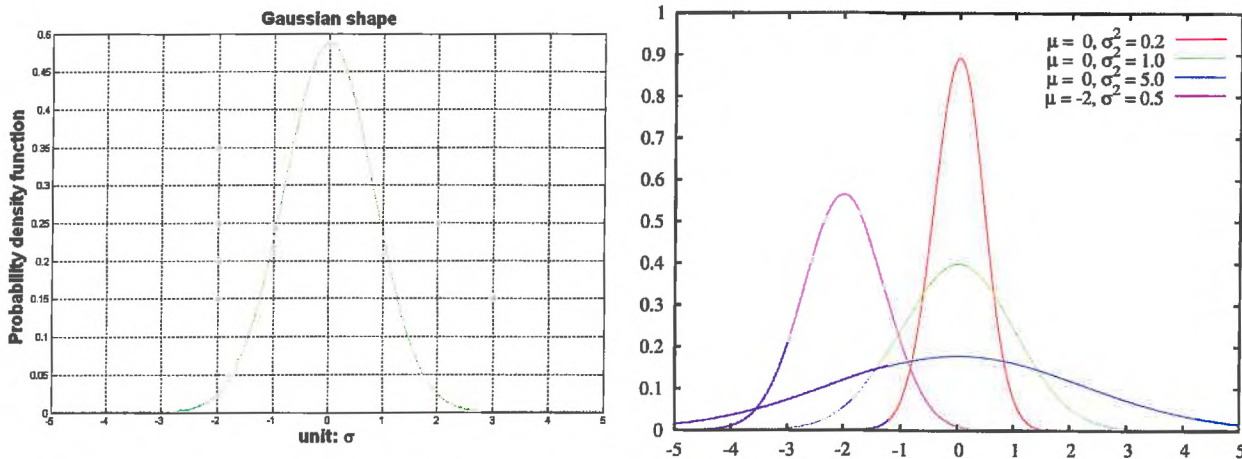
Figure 7 : Courbes de Gauss
