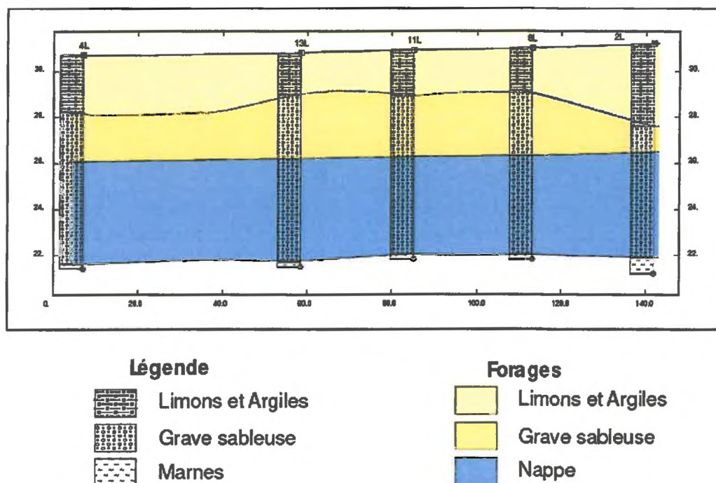
Figure 6 : Coupe géologique en travers du site atelier "Fontanille"
