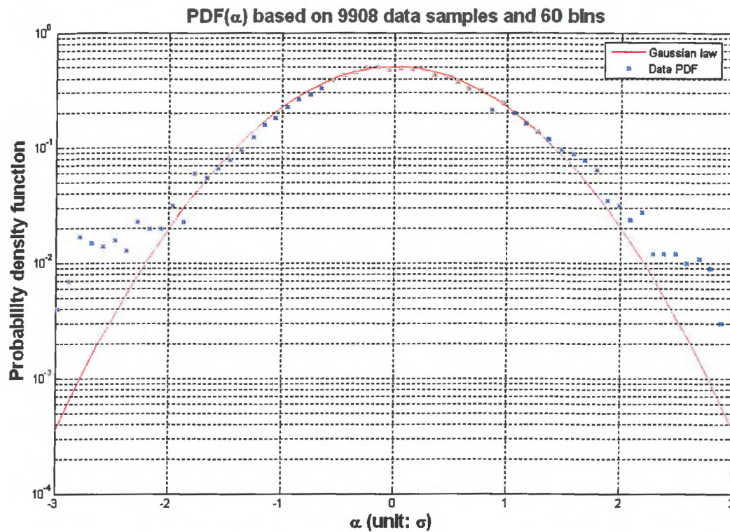
Figure 17 : Log distribution de probabilité des points expérimentaux (en bleu) et log loi normale (en rouge)
