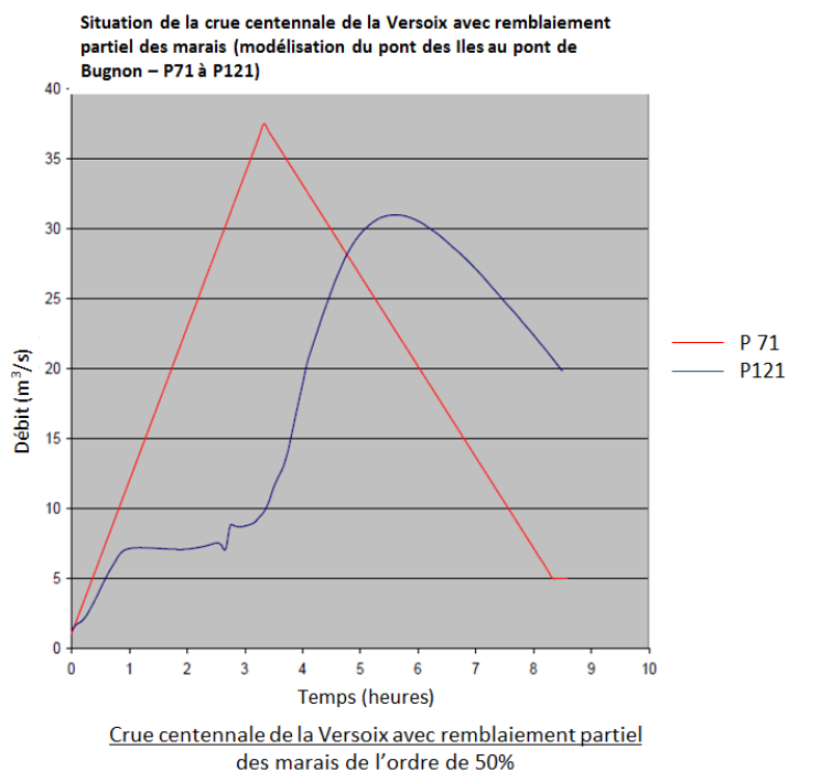
Figure 64 Résultat de la simulation de l'effet des marais de Divonne avec l'hypothèse d'un remblaiement de 50% de la surface du marais (figure extraite de CEN Rhône-Alpes, n.d.)
