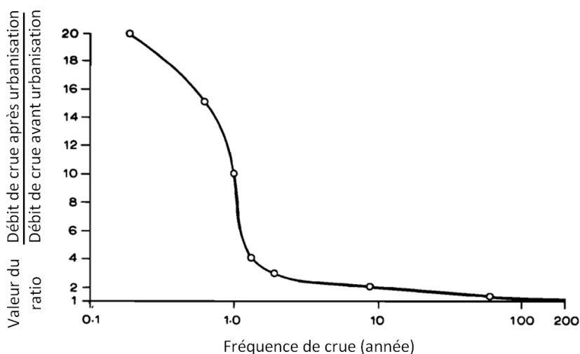
Figure 74 Ratio entre débit de crue après/avant urbanisation en fonction de la fréquence de crue, sur des bassins versants concernés par 20% de surface imperméabilisée (d'après Hollis, 1975)
