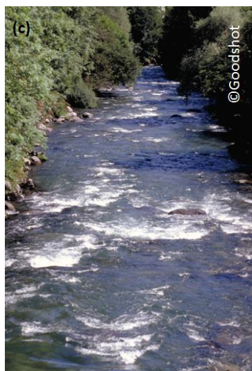
Figure 41 Lit à rapides dans lequel la capacité de transport et la charge solide s'équilibrent
