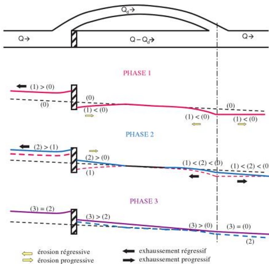
Figure 87 Conséquences morphologiques d'un seuil avec dérivation (figure extraite de Degoutte, 2012)
