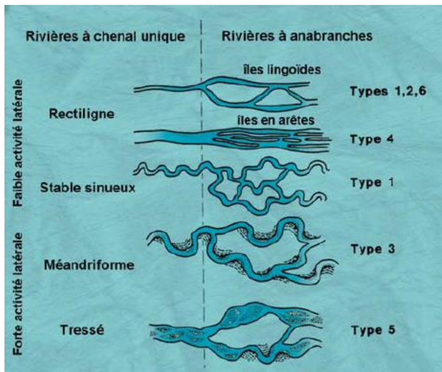
Figure 46 Les différents types de rivières, à chenal unique à gauche et en anabranches à droite (d'après la classification de Nanson et Knighton, 1996, figure extraite de Malavoi et Bravard, 2010).
