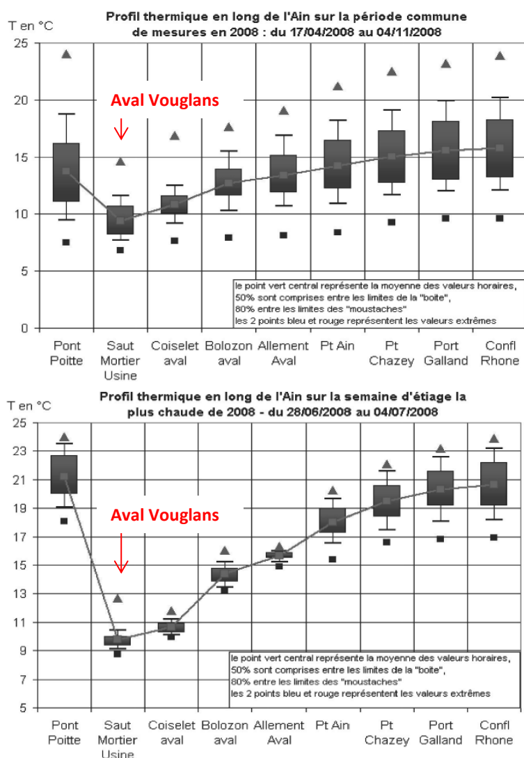
Figure 91 Profils thermiques en long de l'Ain, de l'amont de Vouglans (39) à la confluence avec le Rhône (01) (figure extraite de Poirel et al., 2010)
