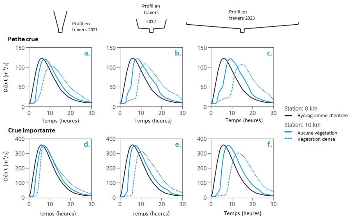
Figure 58 Simulations de la propagation de deux types de crues (faible pour les graphiques a, b et c ; et forte pour les graphiques d, e et f), sur un tronçon de 10km, en fonction de trois types de profil du lit majeur, avec (trait pointillé) ou sans (trait bleu plein) végétation (d'après Brett Anderson, unpublished thesis, modifié d'après Lovett et al., 2007)
