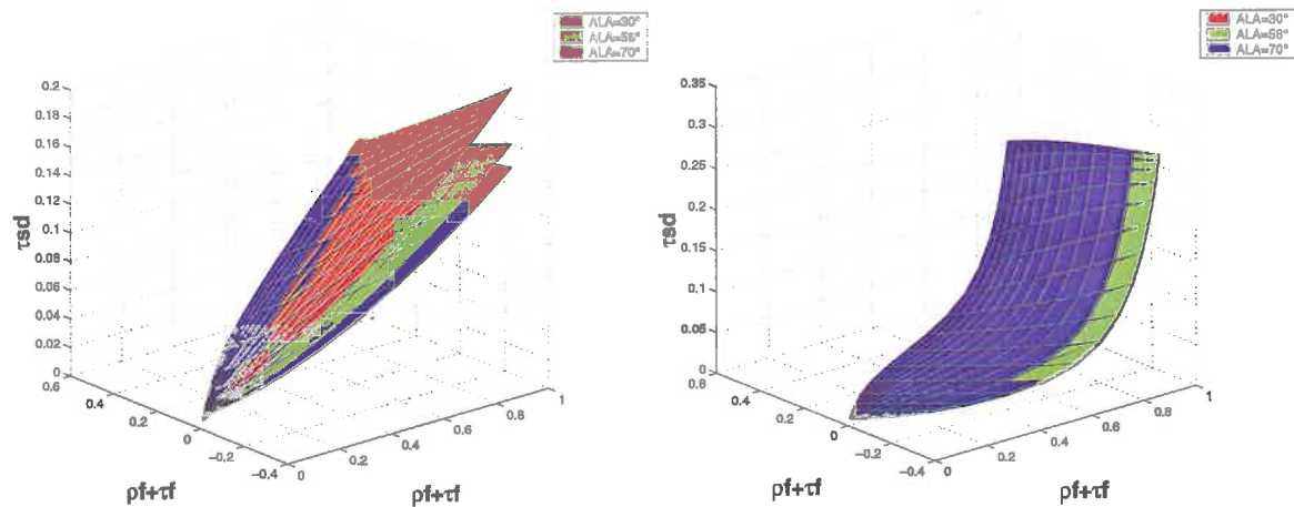
Figure 8 : idem Figure 6 mais pour différents angles moyens d'inclinaisons. ALA=[30^\circ, 58^\circ, 70^\circ] et LAI=0.5 (à gauche) ou 7 (à droite).
