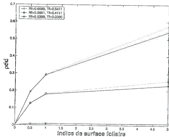
Figure 24 : variation du terme \rho_{dd} en fonction du LAI [0.5 1 5], b/h [0.25 (-), 1(--)], \chi=0 , et les propriétés optiques des feuilles. Les autres caractéristiques sont identiques à celles de la Figure 19
