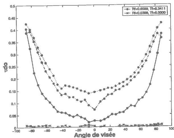
Figure 28 : variation du terme \tau_{do} en fonction de l'angle de visée dans le plan principal, d^* [1(-) 10(-) 100(...)], \chi=0 , et propriétés optique des feuilles. Les autres caractéristiques sont identiques à celles de la Figure 19.
