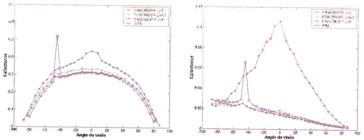
Figure 18 : Comparaison des réflectances simulées par le modèle SAIL et PARCINOPY sur les maquettes 3D. Les caractéristiques des couverts considérées sont : LAI=1 (à droite) 5 (à gauche), \chi=[0 \ 0.5 \ 1] , ALA=58°, b/h=0.25 et d*=100. Les propriétés optiques des feuilles et du sol sont respectivement : \rho_f=0.0398 , \tau_f=0 , \rho_s=1 ; La variation directionnelle est présentée dans le plan principal pour un angle zénithal solaire de -45°.
