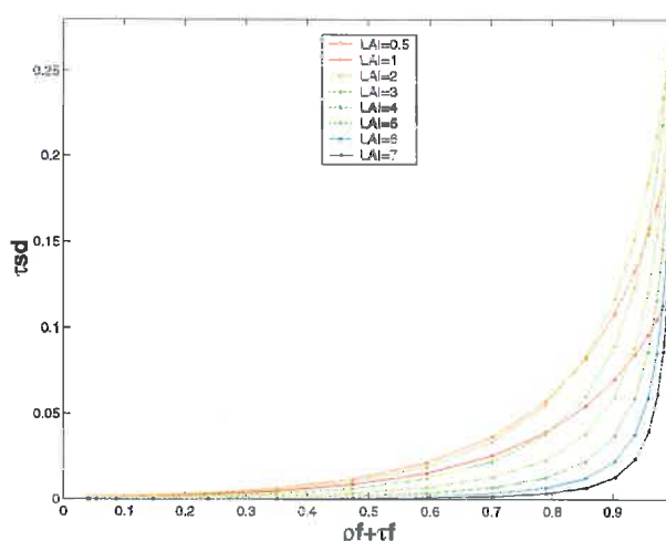
Figure 7 Evolution de la transmittance directionnelle-diffuse du couvert en fonction des propriétés optiques des feuilles et de l'indice de surface foliaire. S^*=0.025 , ALA=30°
