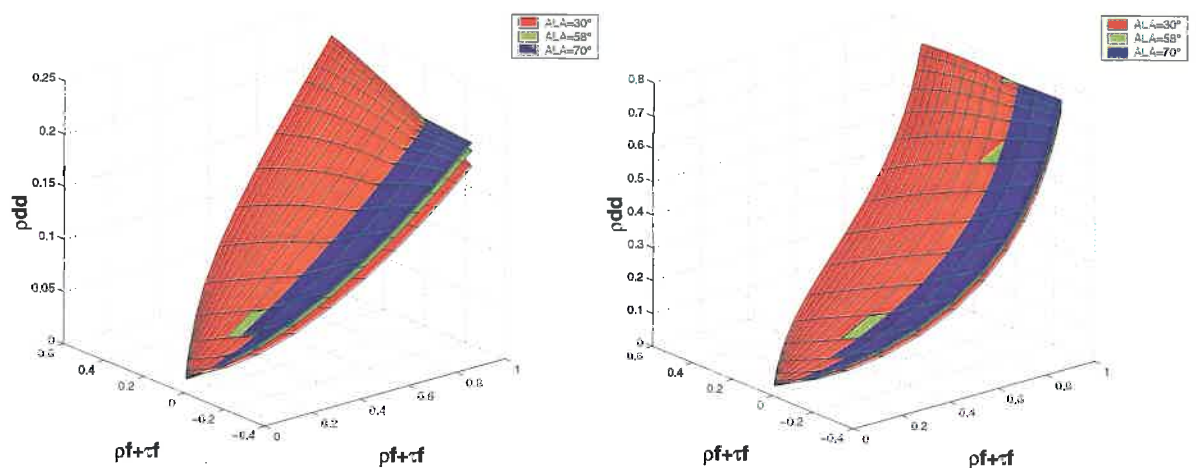
Figure 11 : idem Figure 9 mais ALA=[30°, 58°, 70°] et LAI=0.5 (à gauche) et 7 (à droite).
