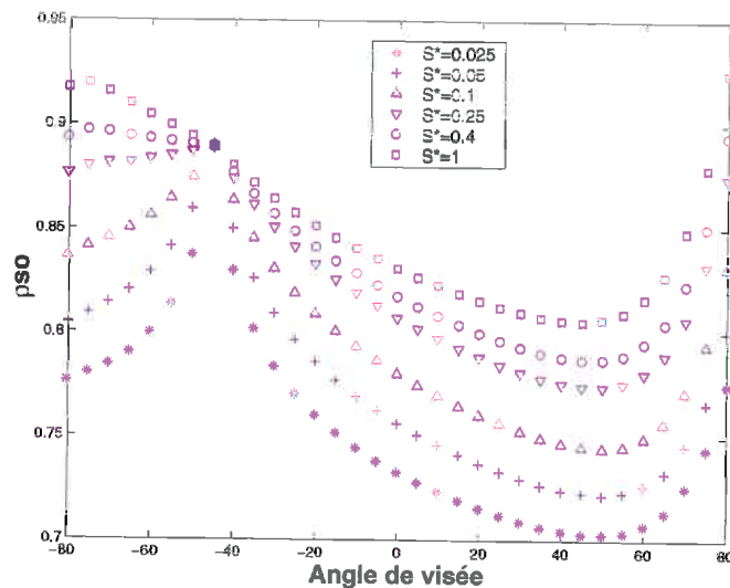
Figure 16 : variation directionnelle dans le plan principal de la réflectance directionnelle-directionnelle en fonction de la taille de la feuille. LAI=7 ; ALA=30^\circ ; \rho_f=0.38 \tau_f=0.62 .
