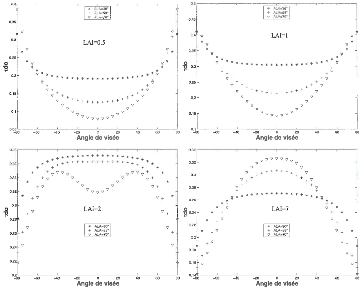
Figure 13 : Variation directionnelle dans le plan principal de la transmittance diffuse-directionnelle en fonction de l'angle moyen d'inclinaison ALA=[30^\circ, 58^\circ, 70^\circ] et du LAI [0.5 1 2 7]. \rho_i=0.38 \tau_i=0.62
