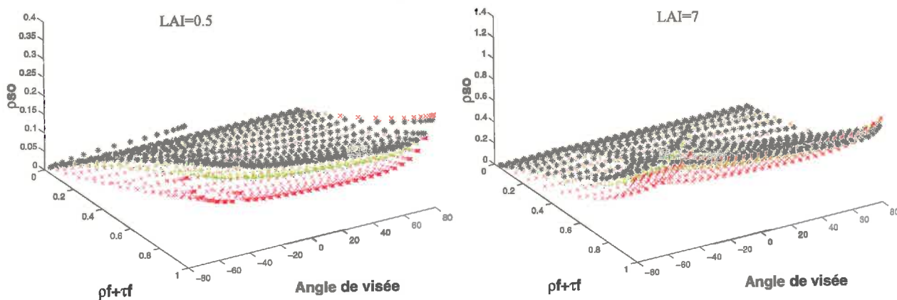
Figure 14 variation directionnelle dans le plan principal de la réflectance directionnelle-directionnelle en fonction de l'albédo de simple diffusion et de trois indices de structure N=[1(\text{rouge}), 2(\text{vert}), 4(\text{noir})] et \text{LAI}=[0.5, 7] , \text{ALA}=30^\circ et S^*=0.025 .
