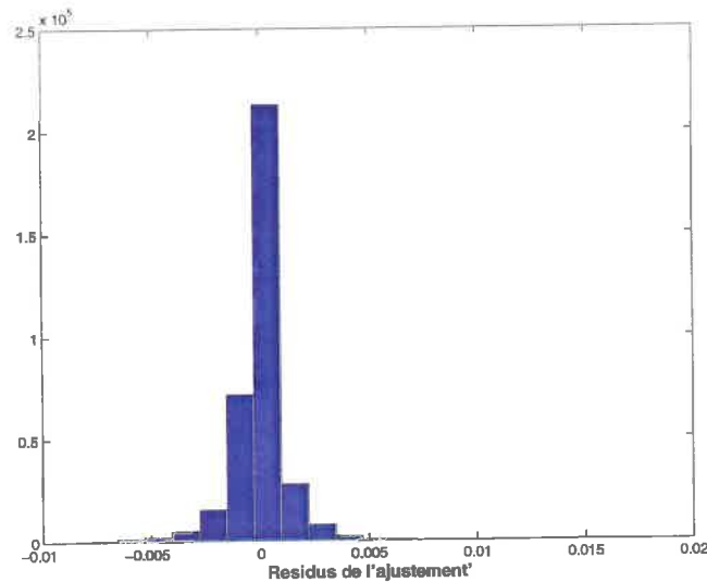
Figure 17 : Distribution des résidus des quatre termes ( \tau_{sd} , \rho_{dd} , \tau_{do} , \rho_{so} ) obtenus par l'ajustement des formalismes ci dessus LAI=[0.5 1 2 3 4 5 6 7], ALA=30° S*=0.025.
