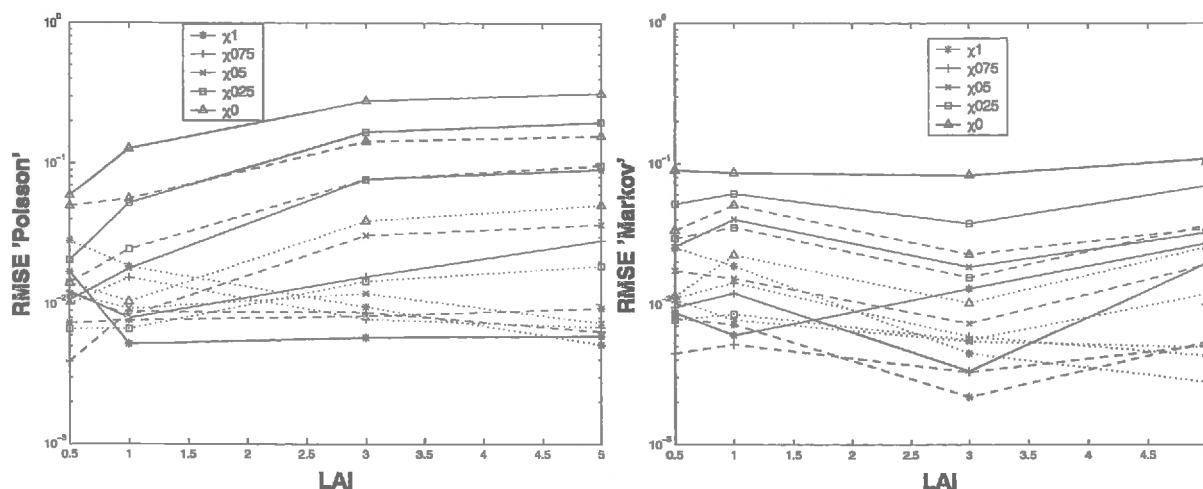
Figure 12 : Exemple de sensibilité à l'indice foliaire de l'erreur quadratique moyenne des deux modèles pour \chi=[0.25 \ 0.5 \ 0.75 \ 1] , S^*=[0.025 \text{ --- } 0.05 \text{ --- } 0.1 \dots] , d^*=100\text{pt} , b/h=0.25 , ALA=58^\circ .
