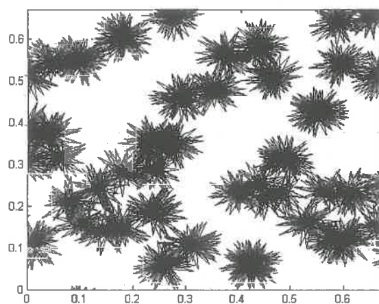
Figure 9 : Vue au nadir des maquettes 3D . Les caractéristiques du couvert considérés sont : LAI=5 , S^*=0.025 , d^*=100 , b/h=0.25 et \chi=[0 \ 0.5 \ 1] .
