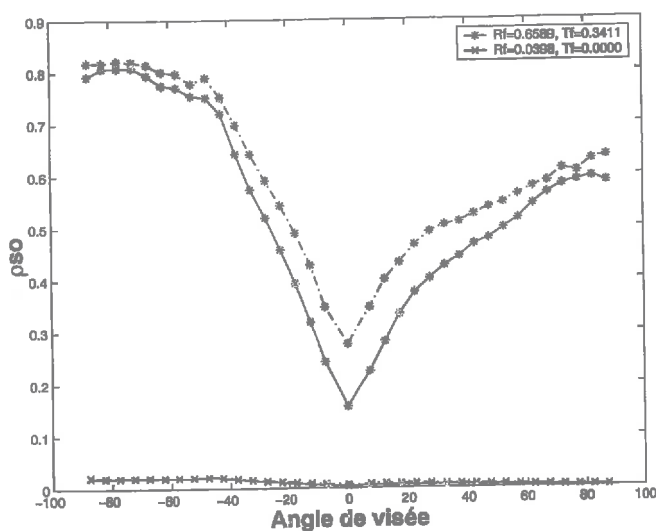
Figure 31 variation du terme \rho_{so} pour un LAI=5 en fonction de l'angle de visée dans le plan principal, b/h [0.25 (-), 1(-.-)], \chi =0, et propriétés optique des feuilles. Les autres caractéristiques sont identiques à celles de la Figure 19.
