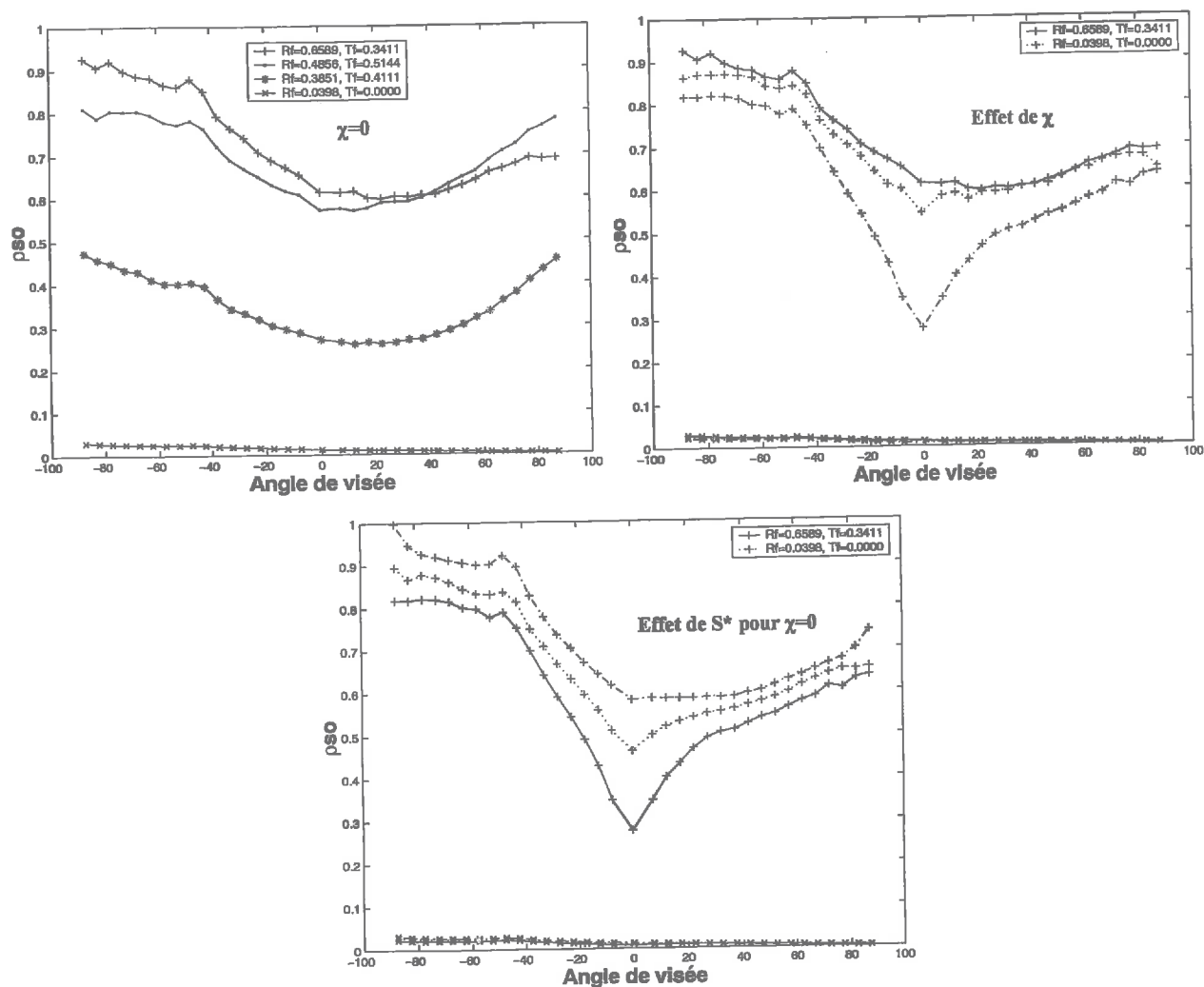
Figure 30 variation du terme \rho_{so} pour LAI=5, en fonction de l'angle de visée dans le plan perpendiculaire, S^* [0.025 (-), 0.05(...), 0.1(-.-)], \chi =[0(-.-), 0.5(...), 1(-)], et propriétés optique des feuilles. Les autres caractéristiques sont identiques à celles de la Figure 19.
