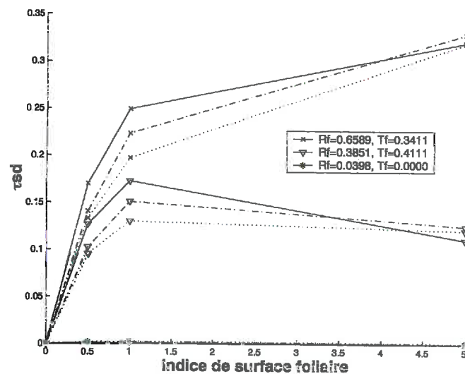
Figure 22 : variation du terme \tau_{sd} , pour \chi=0 , en fonction du LAI [0.5 à 5], ALA [30° (-), 58° (--), 70° (....)] et les propriétés optiques des feuilles. Les autres caractéristiques sont identiques à celles de la Figure 19.
