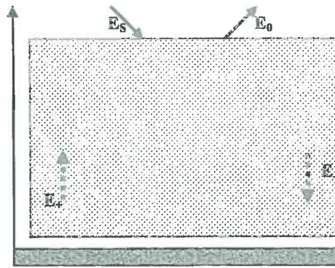
Figure 5 : schéma des flux dans un modèle turbide monocouche.
