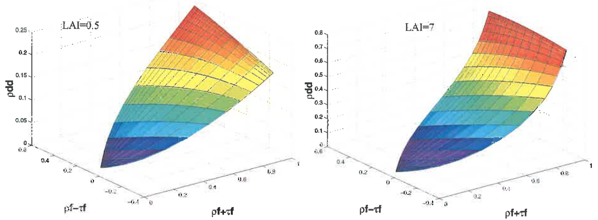
Figure 9 Variation de la réflectance diffuse-diffuse en fonction de l'albédo de simple diffusion et de la différence entre la réflectance et la transmittance de la feuille pour plusieurs LAI [0.5 7] et ALA=30°.
