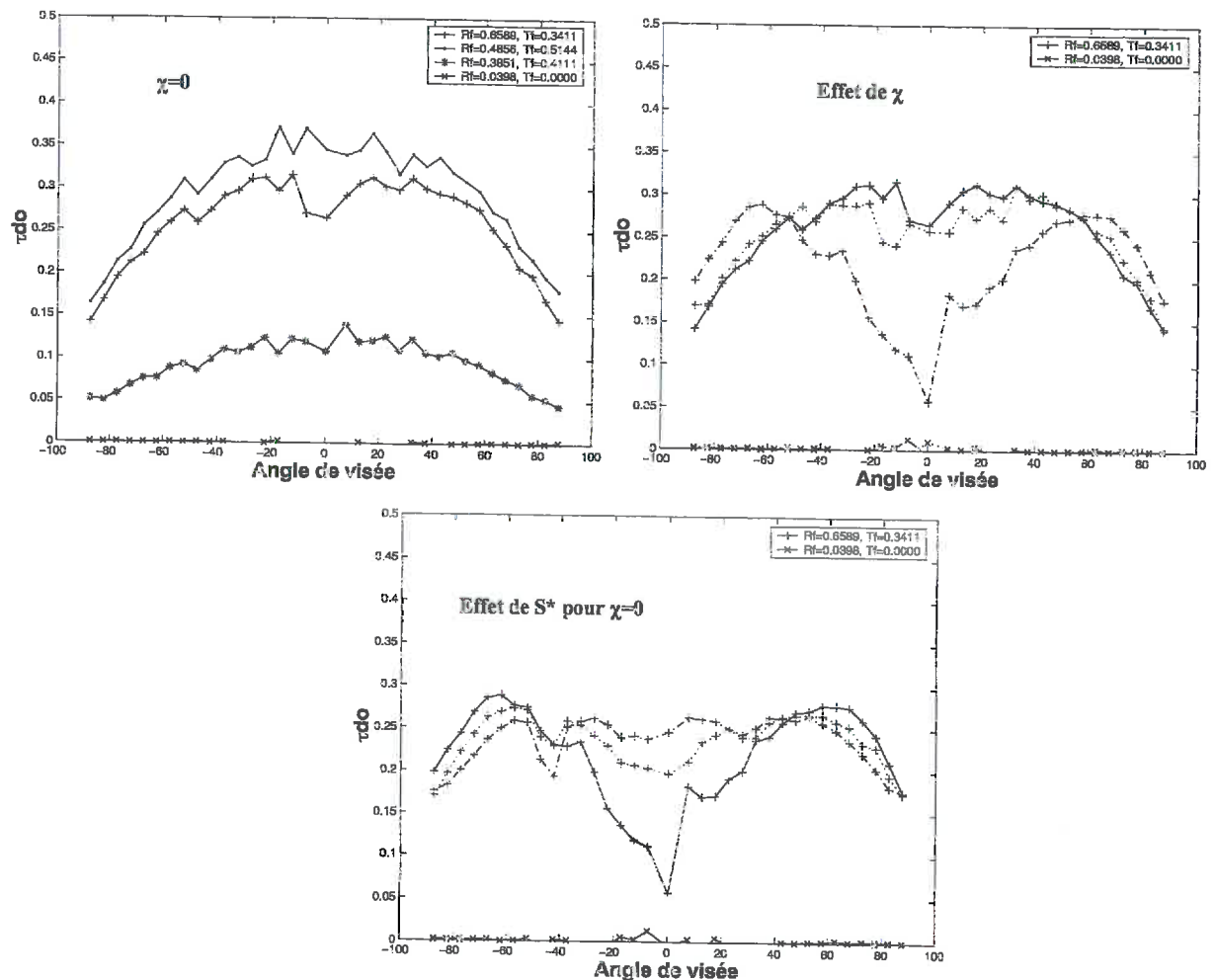
Figure 26 : variation du terme \tau_{do} pour LAI=5, en fonction de l'angle de visée dans le plan perpendiculaire, S^* [0.025 (-), 0.05(...), 0.1(-.-)], \chi =[0(-.-), 0.5(...), 1(-)], et propriétés optiques des feuilles. Les autres caractéristiques sont identiques à celles de la Figure 19.
