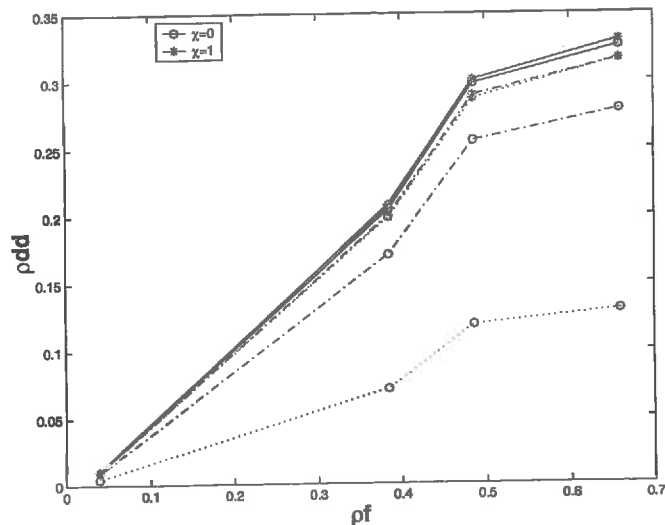
Figure 25 : variation du terme \rho_{dd} en fonction de la densité des plantes, d^* [1(...) 10(—) 100(-)], et la réflectance des feuilles. LAI=1, S^*=0.1 , ALA=58°. Les autres caractéristiques sont identiques à celles de la Figure 19
