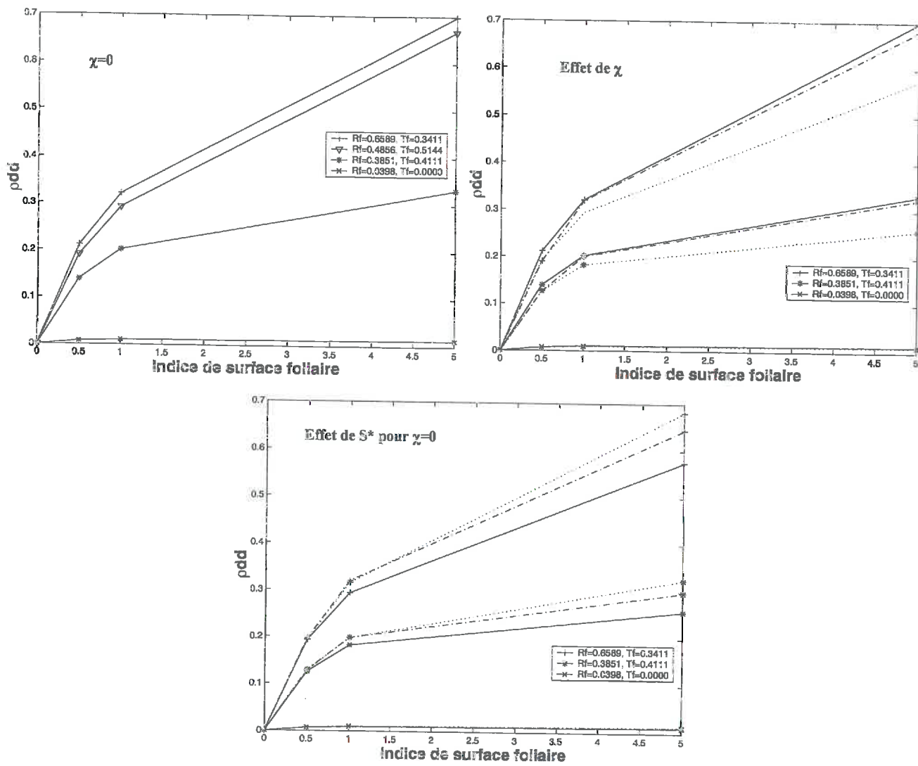
Figure 23 : variation du terme \rho_{dd} en fonction du LAI [0.5 1 5], S^* [0.025 (-), 0.05(-), 0.1(...)], \chi =[0(...), 0.5(--), 1(-)], et les propriétés optiques des feuilles. Les autres caractéristiques sont identiques à celles de la Figure 19
