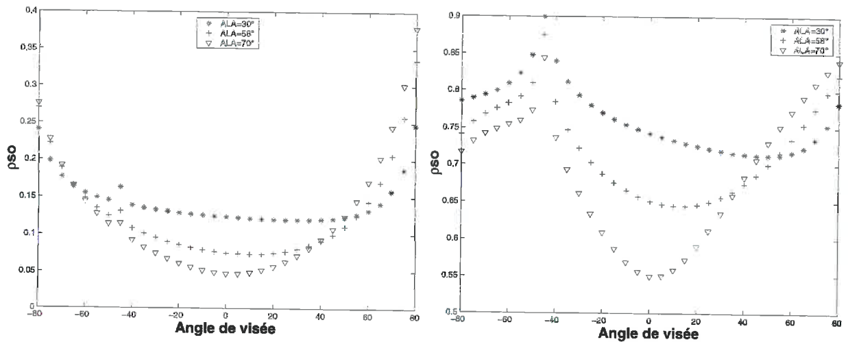
Figure 15 : variation directionnelle dans le plan principal de la réflectance directionnelle-directionnelle en fonction des angles moyens d'inclinaisons ALA=[30^\circ, 58^\circ, 70^\circ] et du LAI=0.5 (à gauche) et 7 (à droite) S^*=0.025 et \rho_f=0.38 \tau_f=0.62 .
