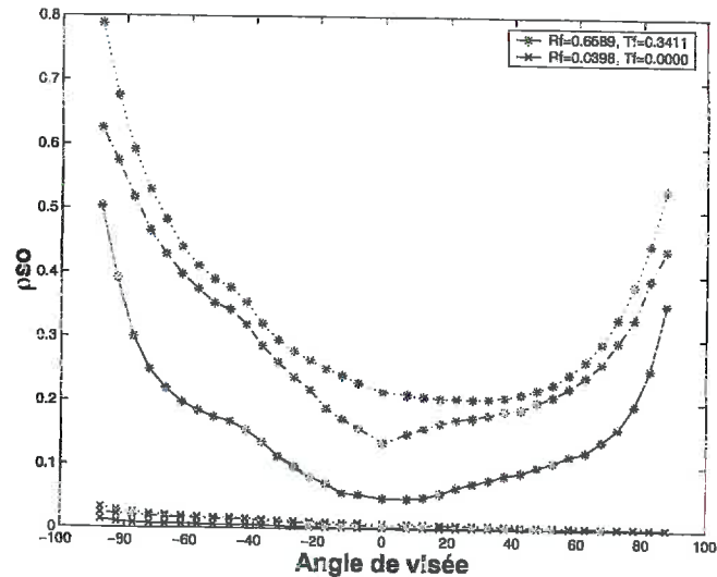
Figure 32 variation du terme \rho_{so} en fonction de l'angle de visée dans le plan principal, d^* [1(-) 10(-- ) 100(...)], \chi=0 , et propriétés optiques des feuilles. Les autres caractéristiques sont identiques à celles de la Figure 19.
