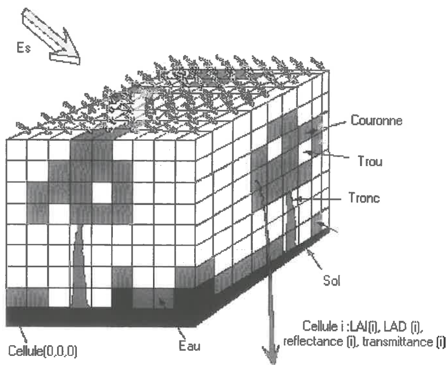
Figure 6 : schéma descriptif de la discrétisation dans le modèle DART (Gastellu-Etchegorry, Demarez et al. 1996)
