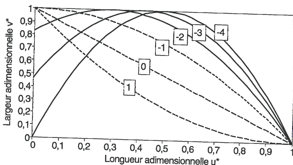
FIG. 1.3 - Modèle de forme de la feuille développée. Le modèle permet de définir différentes formes de la feuille développée, selon la valeur du paramètre \alpha (la représentation est faite en coordonnées adimensionnelles u^* = u/u_f et v^* = v/v_f ).
