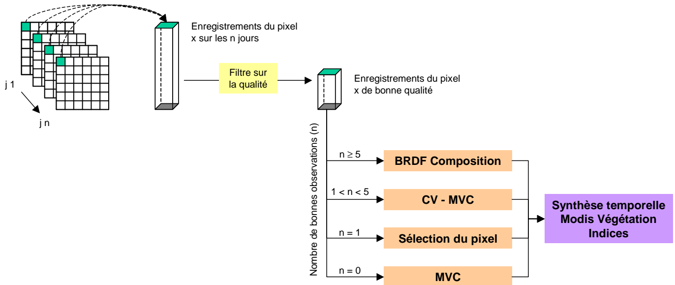
Figure 5 : Algorithme pour la constitution des synthèses temporelles des indices de végétation MODIS
