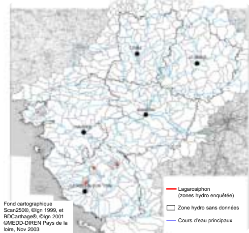
Carte de répartition du Lagarosiphon en Pays de la Loire en 2002.
