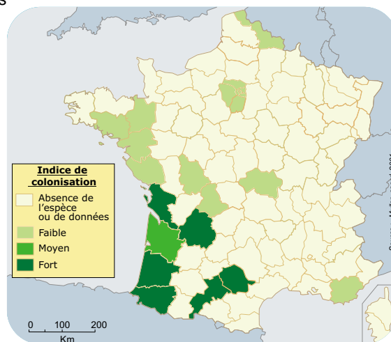
Carte de répartition du Lagarosiphon en France (2002)
