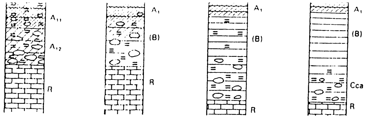
Rendzine brunifiée
