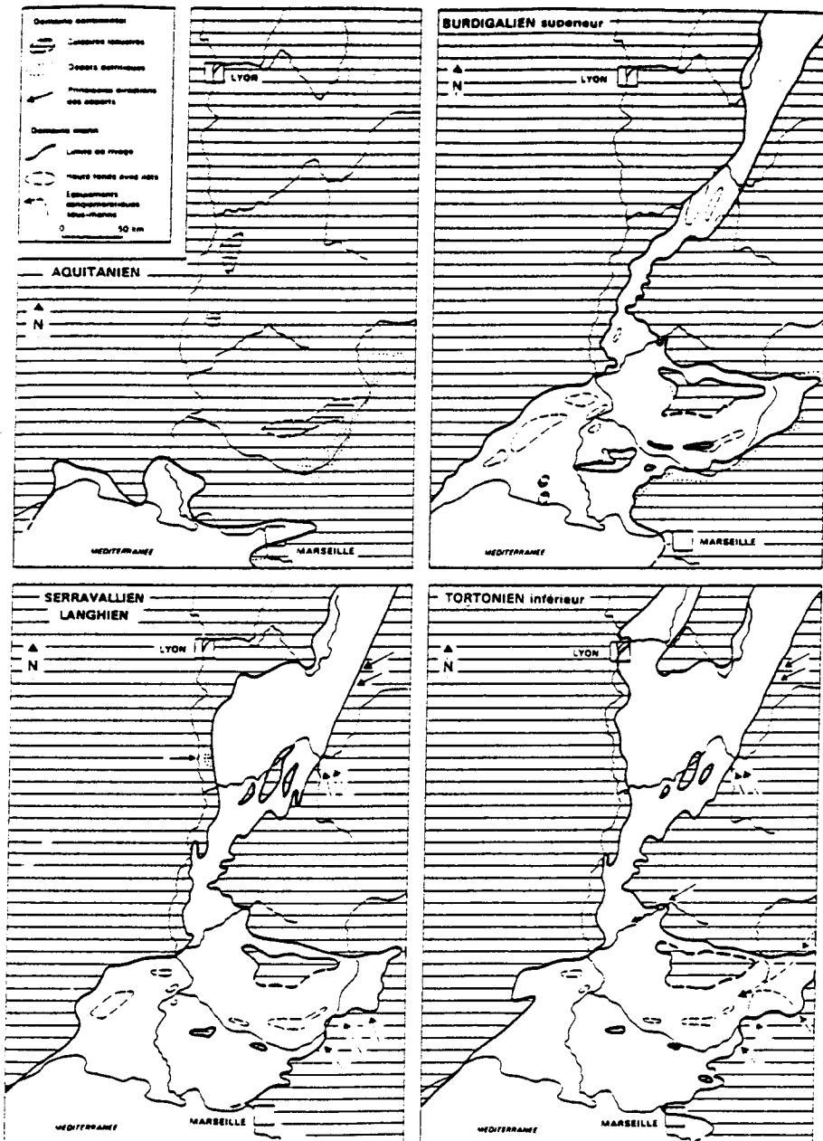
Reconstitution de la paléogéographie du Sud-Est de la France, de l'Aquitainien au Tortonien (BRGM, 1984, p. 505)
