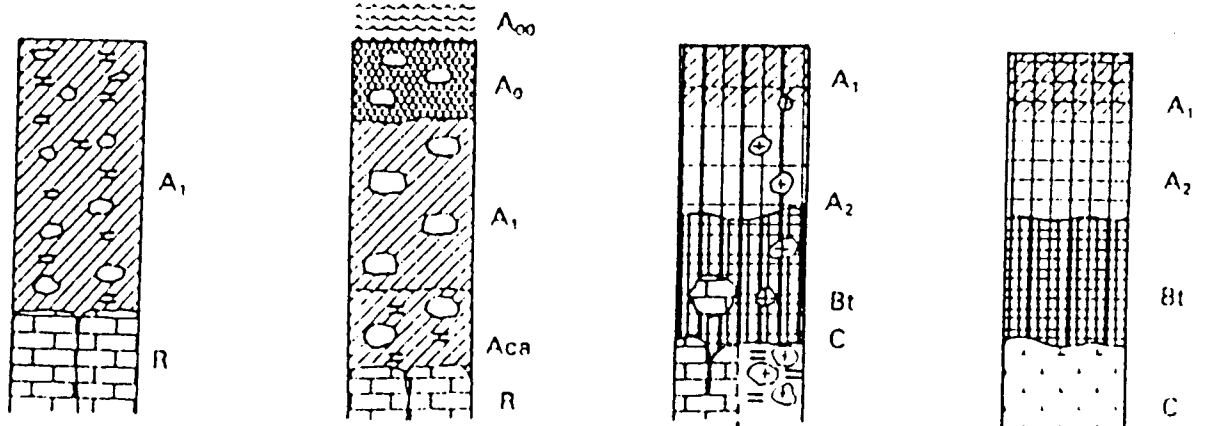
Sol rouge fersiallitique
