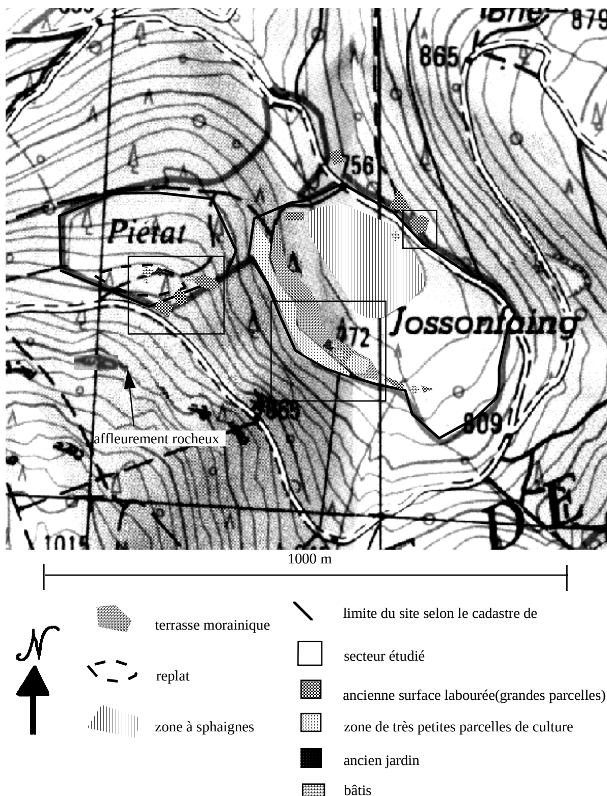
Figure 16 Les sites du Jossonfaing et du Piétal (extrait de la carte IGN Top 25 3618 OT)
