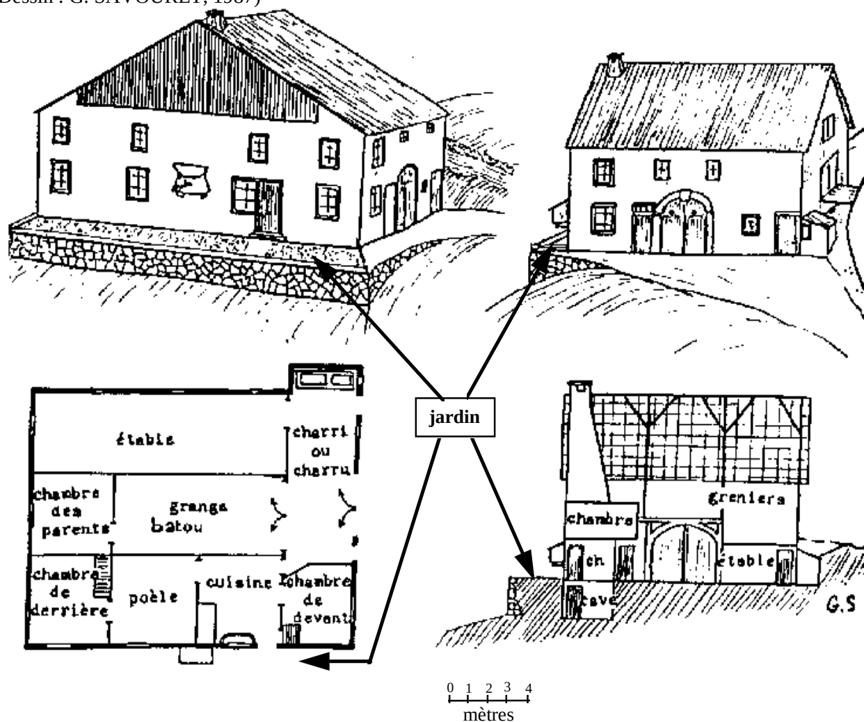
Figure 2-5 Type de jardin étudié - replat artificiel
