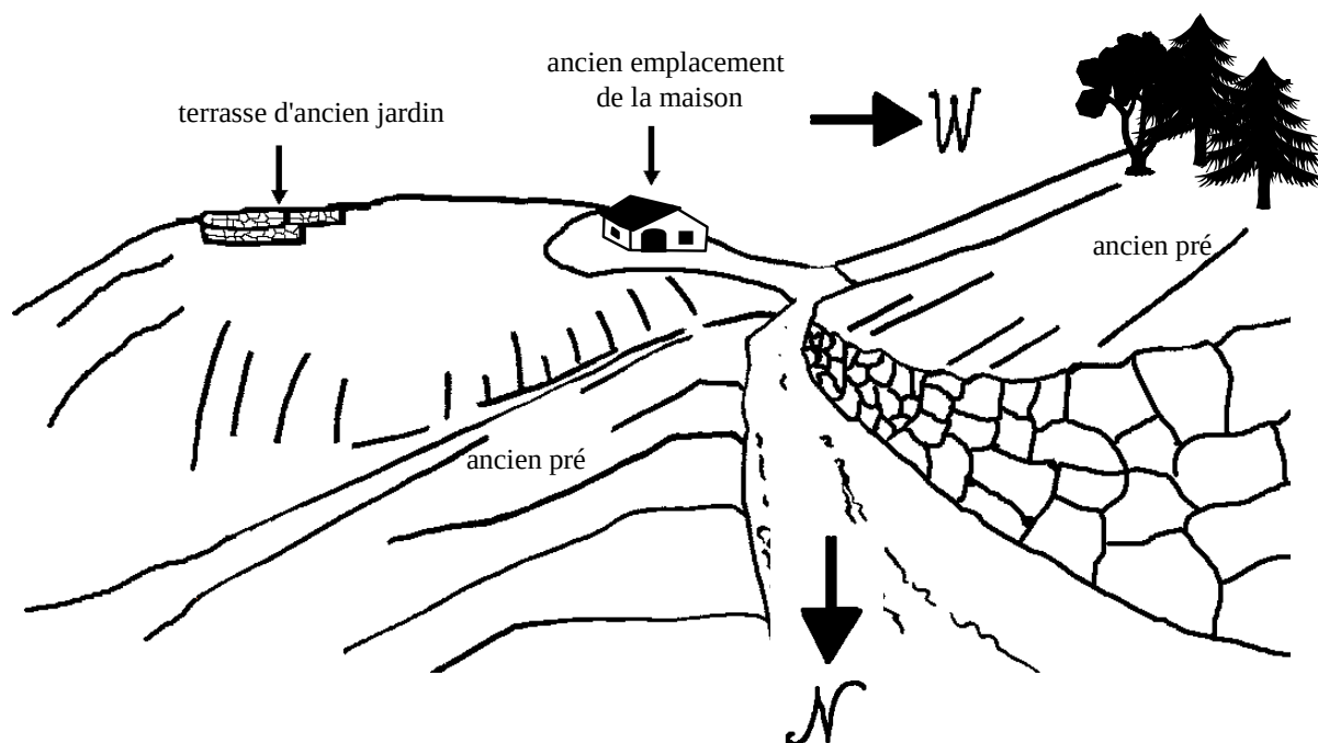
Figure 15 Le site de la Haniroche en limite de la paroi de la niche
