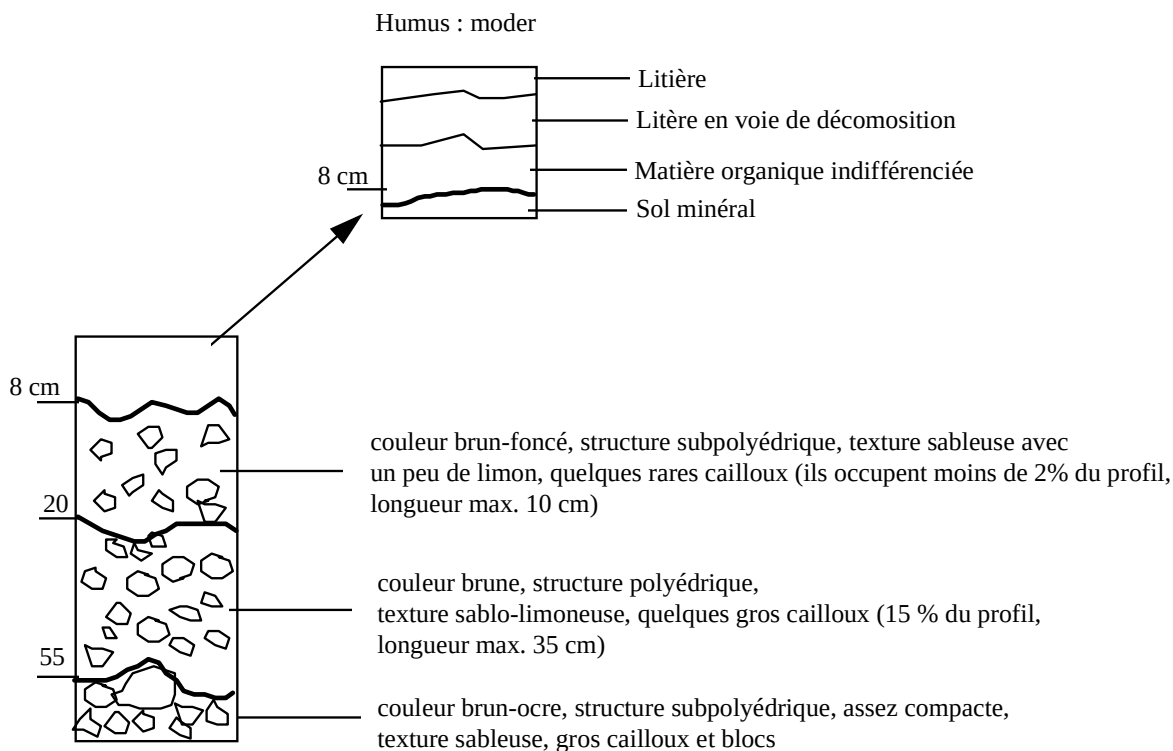
Figure 3-2 Exemple d'un profil pédologique d'un sol brun ocreux à la Pissière
