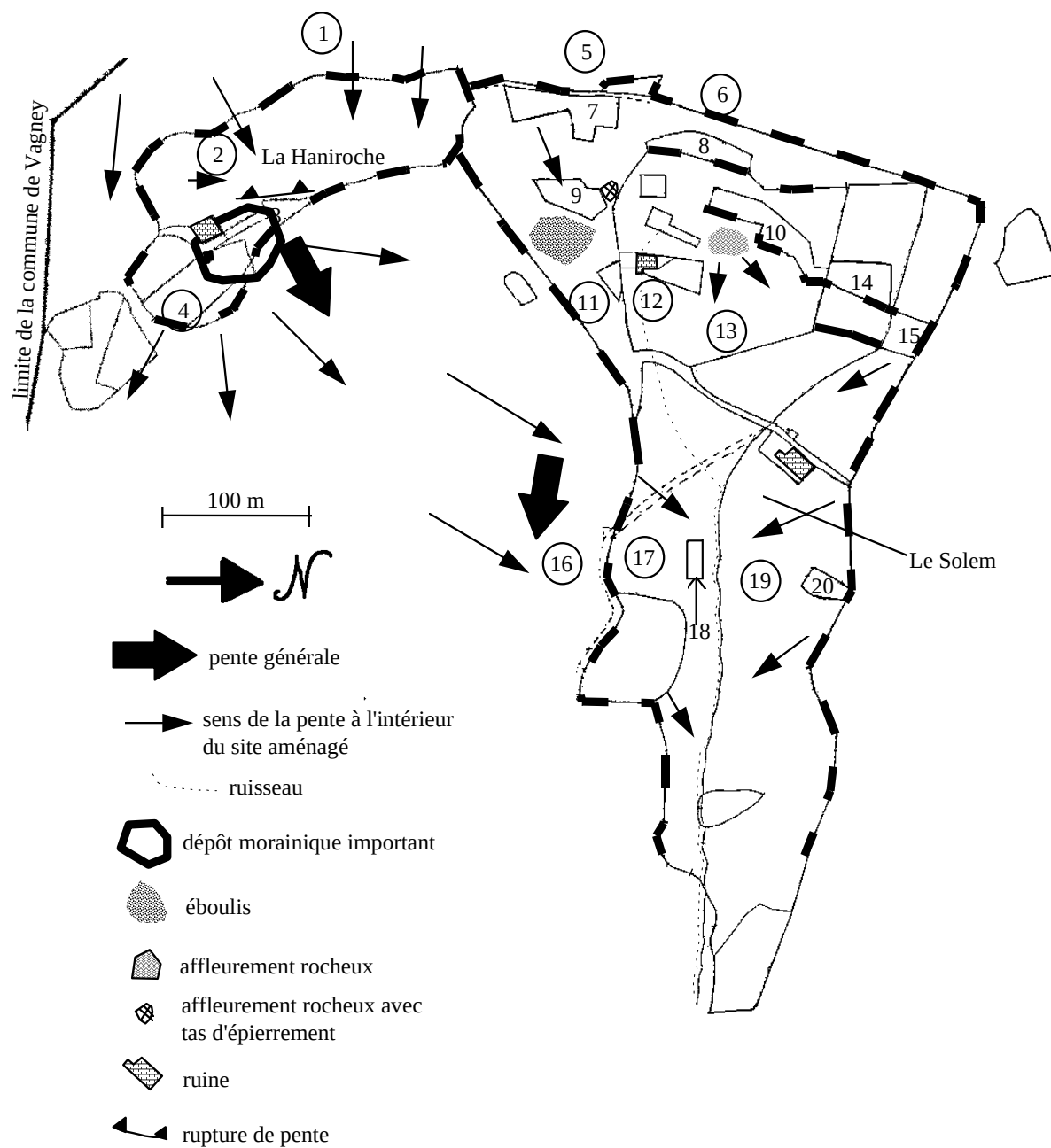
Figure 12 Le Solem et la Hanicroche, schéma géomorphologique et plan cadastral de 1835
