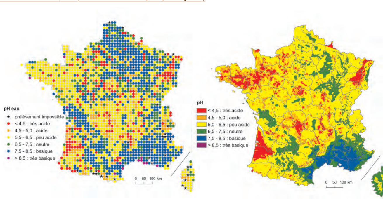
Le pH des horizons de surface des sols de France métropolitaine des sites du Réseau de Mesures de la Qualité des Sols (mesuré) et celui des sols forestiers (prédit par la végétation)
